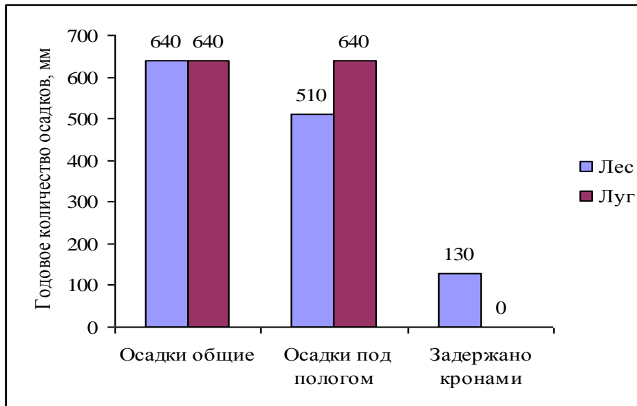
Рис. 1. Распределение осадков в лесу и на лугу
