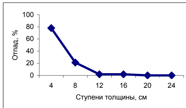
Рис. 2. Зависимость процента отпада от диаметра древостоя
